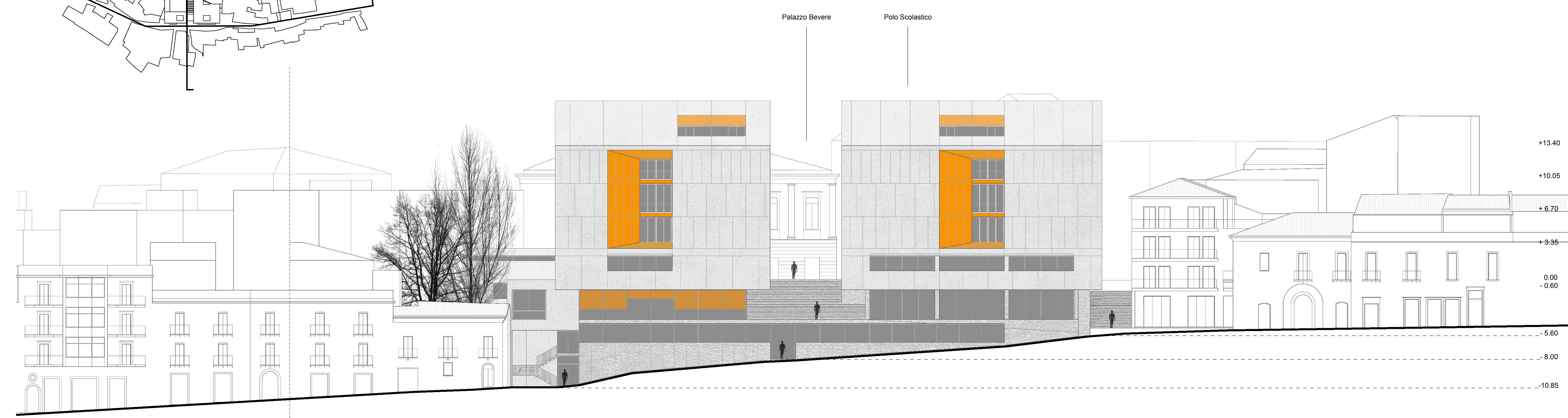
PROFILO AA' SU VIA D'AFFLITTO, scala 1:200
