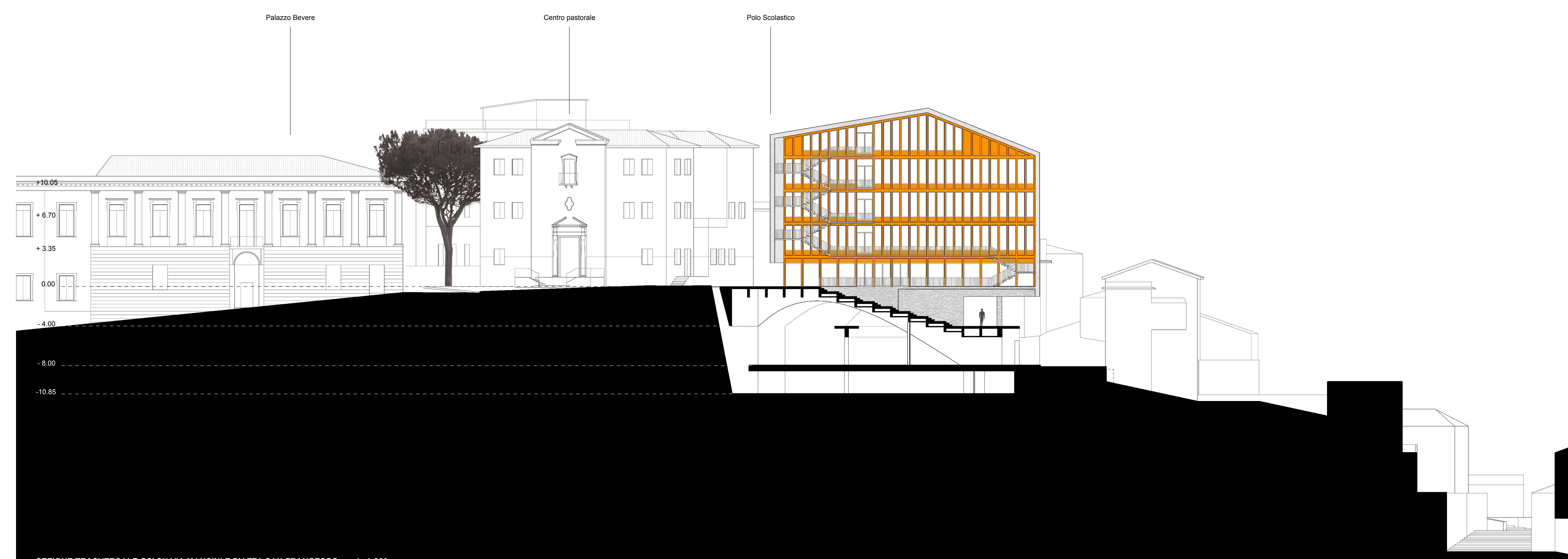
SEZIONE TRASVERSALE CC' SU VIA MANCINI E PIAZZA SAN FRANCESCO, scala 1:200
